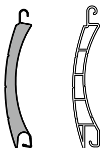
Lame Alu ou Lame PVC Choix d'un tablier PVC ou Alu
