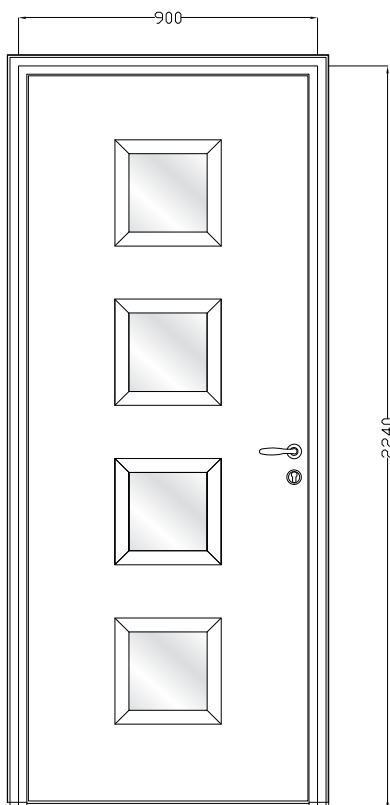
OCTOPUS COMPOSÉE DE 4 VITRAGES EN SUR-MESURE
