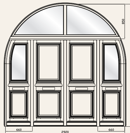
Réalisation du design d'une porte alu (odyssée) adaptée au projet du client avec semi fixes cintrés en partie haute.
